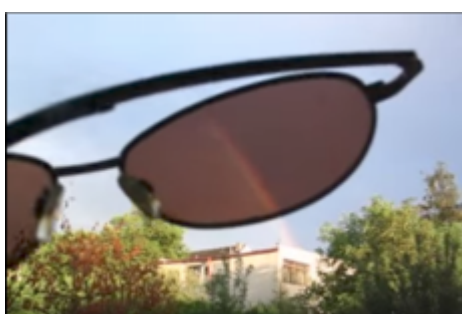
Figura 3. Polarización del arco iris
