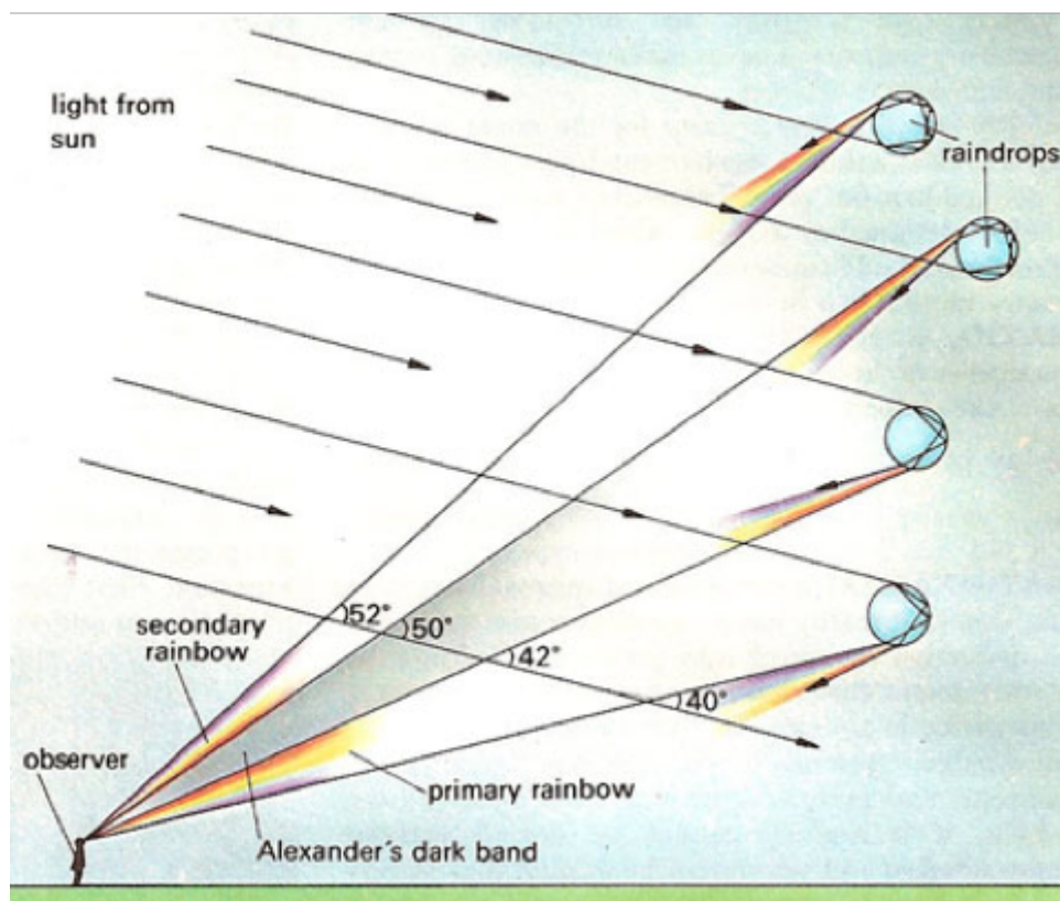
Figura 2. Origen de los dobles arco iris y de la banda de Alexander .
