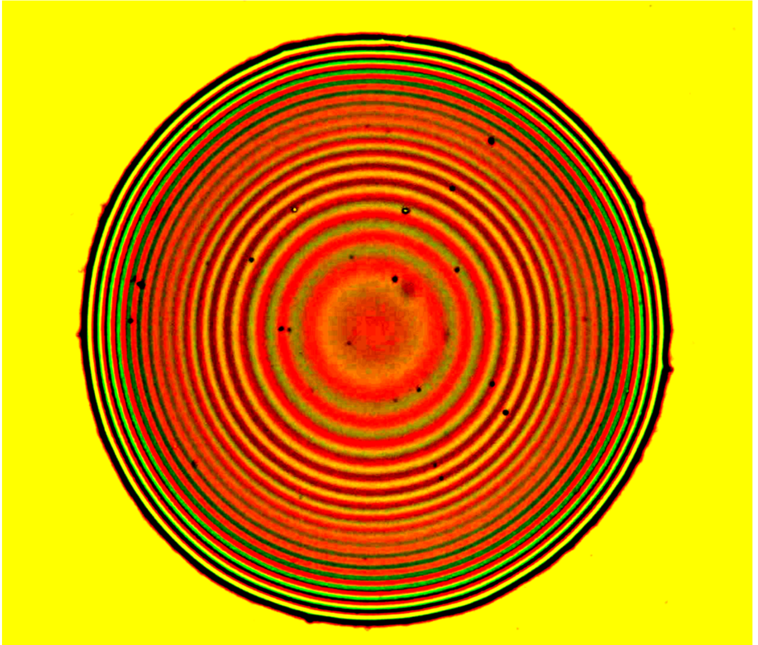
Figura 6. Gota de polidimetilsiloxano (PDMS) de aproximadamente 1 \times 10^{-12} L. Los anillos se generan
