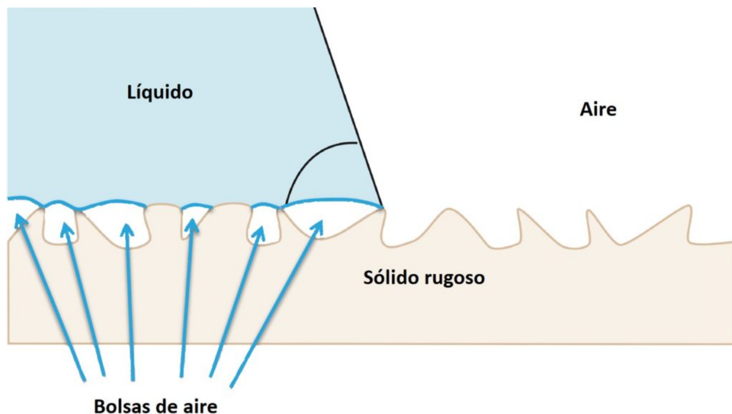
Figura 5. Modelo de Cassie-Baxter.
