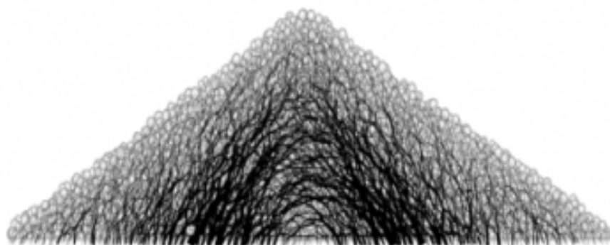
Figura 7. Cadenas de fuerzas en un modelo discreto de pilas de arena .
