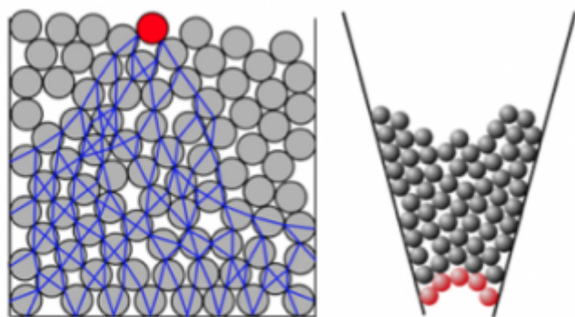
Figura 6. (a) Cadena de transmisión del estrés (nótese
