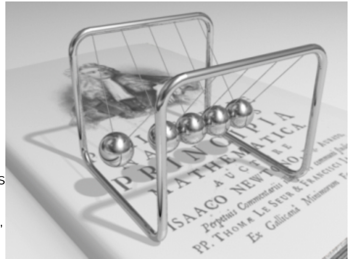
Mecánica newtoniana
